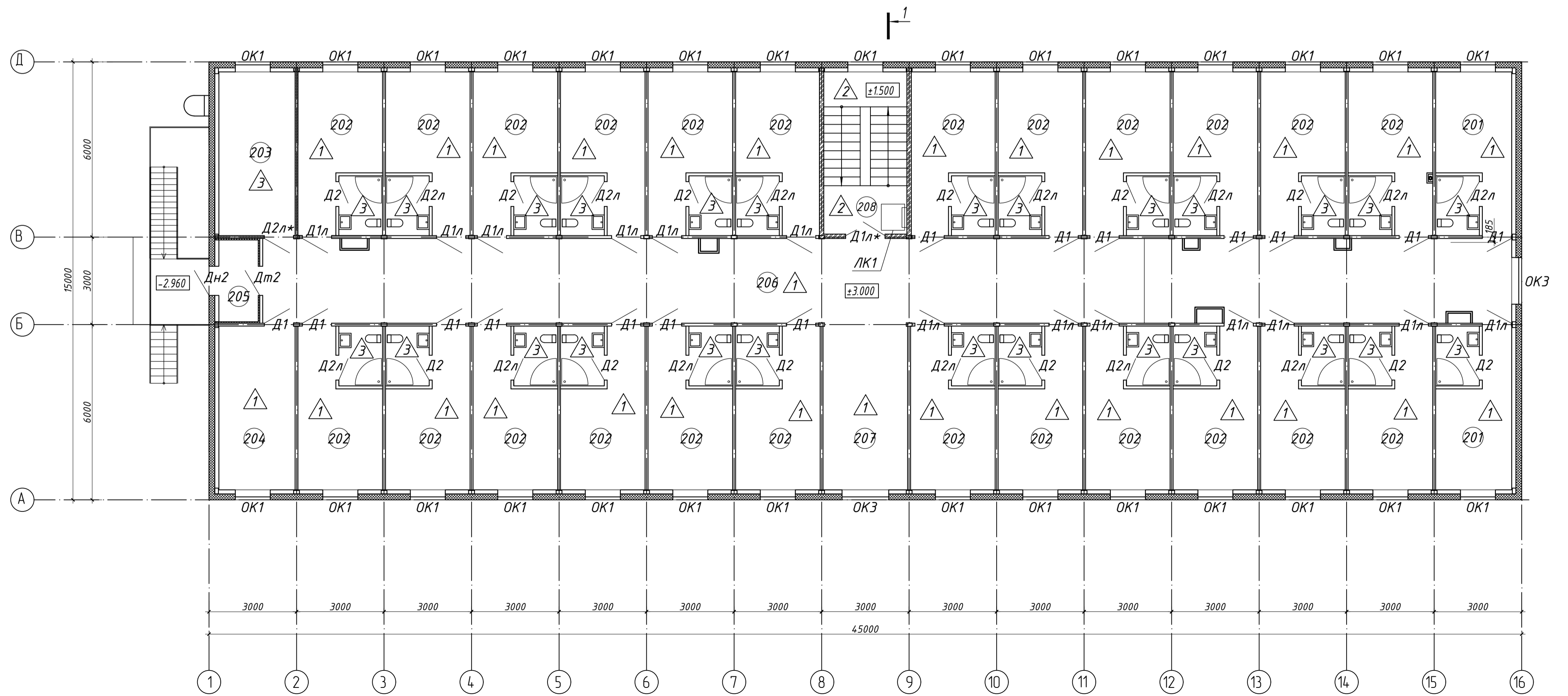
План на отм. +3.000
